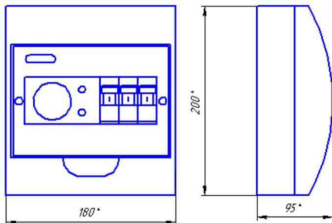
Рисунок 2 – Габаритные размеры изделия
