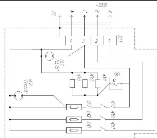
Схема электрическая принципиальная.
